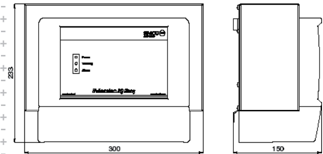
Technische tekening Extension IQ Easy
